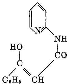
LXIII
